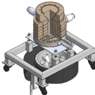
ADSD Modular Die
